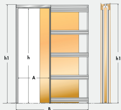
SYSTEM CLASSIC ΣΥΡΟΜΕΝΗ ΧΩΝΕΥΤΗ ΠΟΡΤΑ ΜΕ ΞΥΛΙΝΗ ΚΑΣΑ
