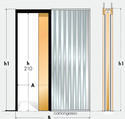
SYSTEM NODOOR ΣΥΡΟΜΕΝΗ ΧΩΝΕΥΤΗ ΠΟΡΤΑ ΧΩΡΙΣ ΞΥΛΙΝΗ ΚΑΣΑ
